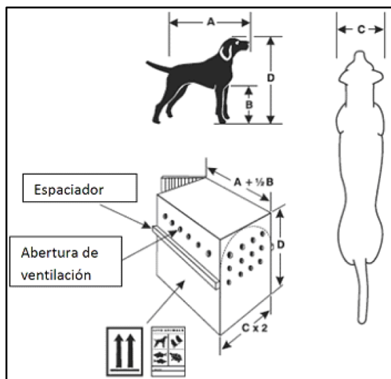
Características de la transportadora para viajes en avión de animales domésticos. Diario Oficial de la Federación.
